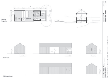
Grundriss neue Schihütte
